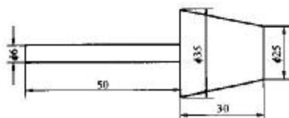
图1 磨光头加工示意图
